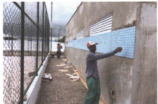
INSTALAÇÃO DO REVESTIMENTO CERÂMICO EXTERNO DOS VESTIÁRIOS DAS QUADRAS
